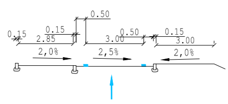
Lõige 2-2 M 1:200
